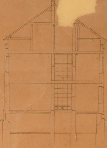
Lunzschnitt nach c. d.
